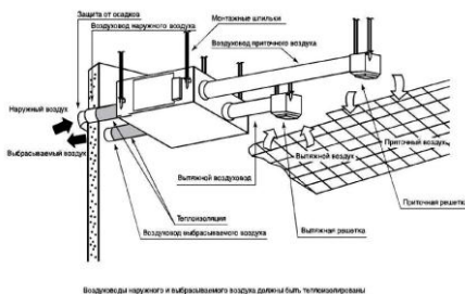
Воздуховоды наружного и выбрасываемого воздуха должны быть теплоизолированы
